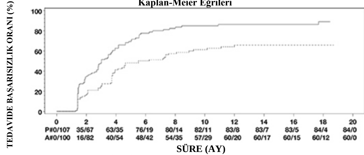
Şekil 2. 6. Hafta veya Sonrasında (UV I Çalışması ) ya da 2. Hafta veya Sonrasında (UV II Çalışması) Tedavide Başarısızlık Ortaya Çıkana Kadar Geçen Süreyi Özetleyen Kaplan-Meier Eğrileri
