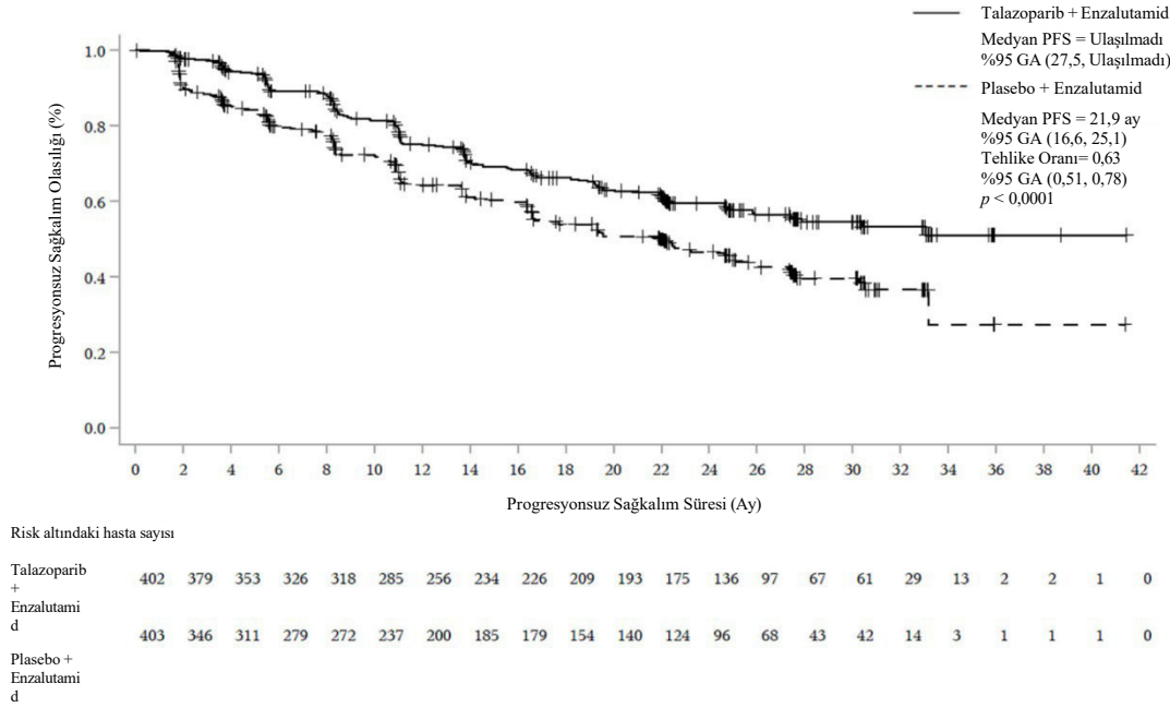
Şekil 1. BICR ile rPFS Kaplan-Meier eğrileri — TALAPRO-2 (mCRPC)
